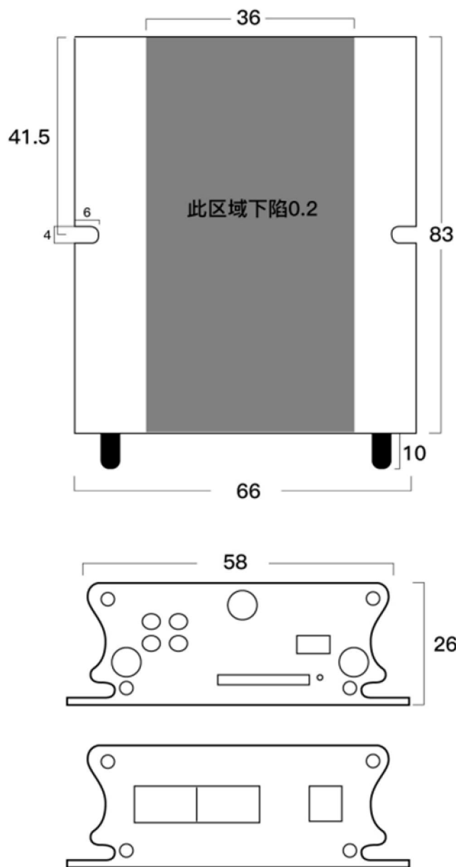
外壳定位孔示意图 (mm)
